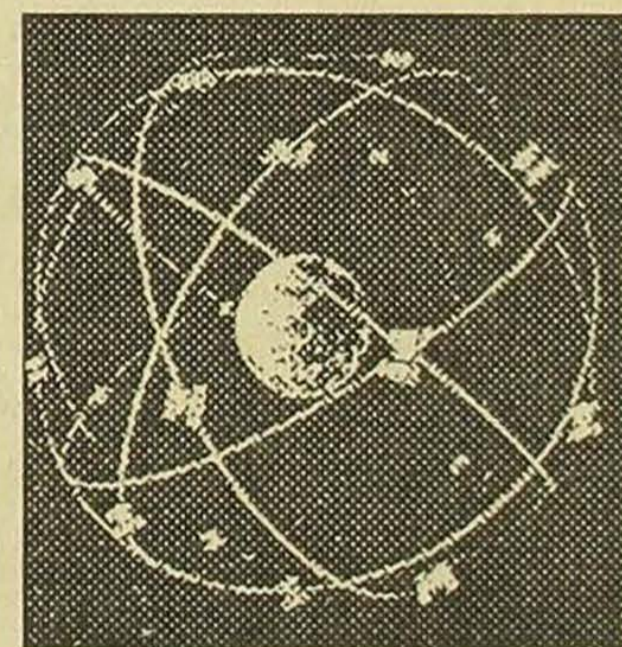
GPS sateliti u svojim orbitama
