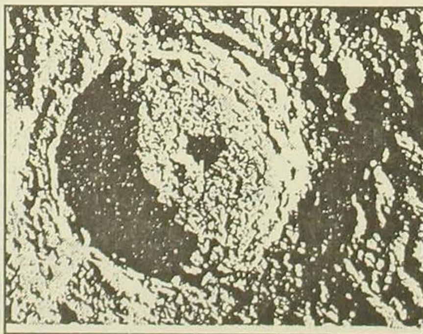
Detalj površine Mjeseca snimljen iz svemirskog broda
