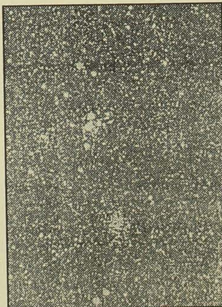
Rasijani zvjezdani skupovi M 46 i M 47 u sazviježdu Pupis
