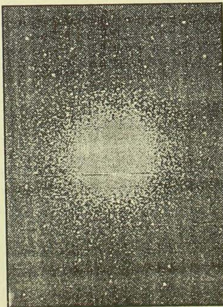
Kuglasti zvjezdani skup M 13 u sazviježdu Herkul
