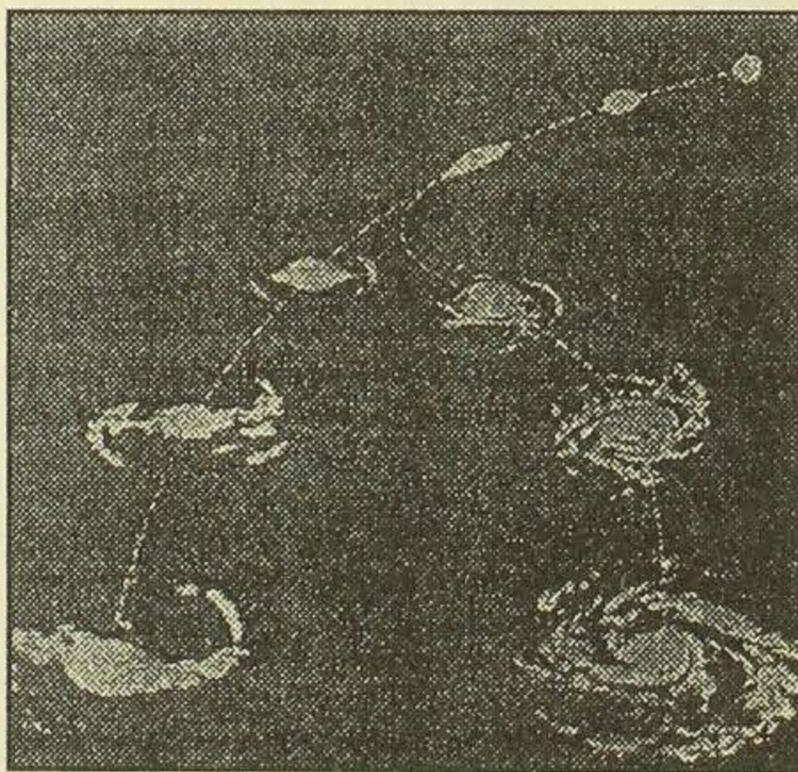
Klasifikacija galaksija. Gornji niz su eliptičke galaksije, koje se granaju na dvije glavne grupe spiralnih
